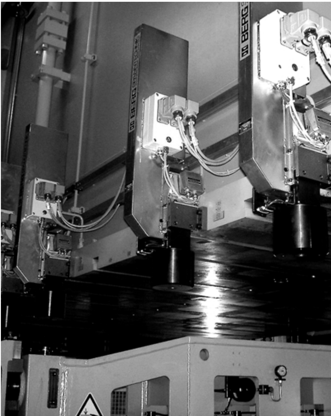
Anwendungsbeispiel Typ PSP...T/PSV-ASI
