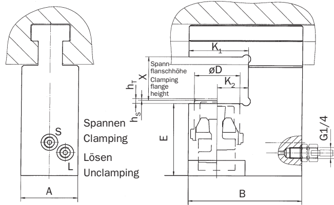
T-Nut nach Kundenangabe T-slot customized
